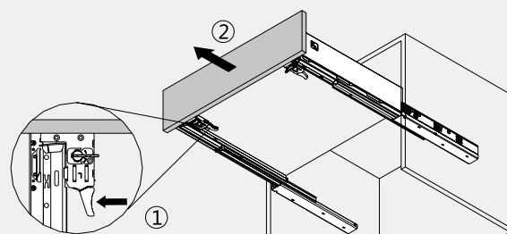
Extracción cajón
