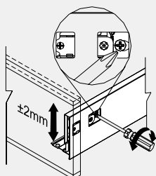
Ajuste altura
