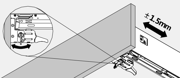
Ajuste profundidad
